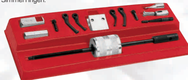
CJ93B Universeller Abziehersatz. 2-armig mit Konterschlaggewicht für Innen- und Außenlager. Reichweite bis zu 63mm, Innendurchmesser 9.53 - 31.75mm, Außendurchmesser bis zu 76mm. Ideal für Nadellager und mit Ausdreheraufnahme und Schlaggewicht ideal zum Ausziehen von Simmerringen.
